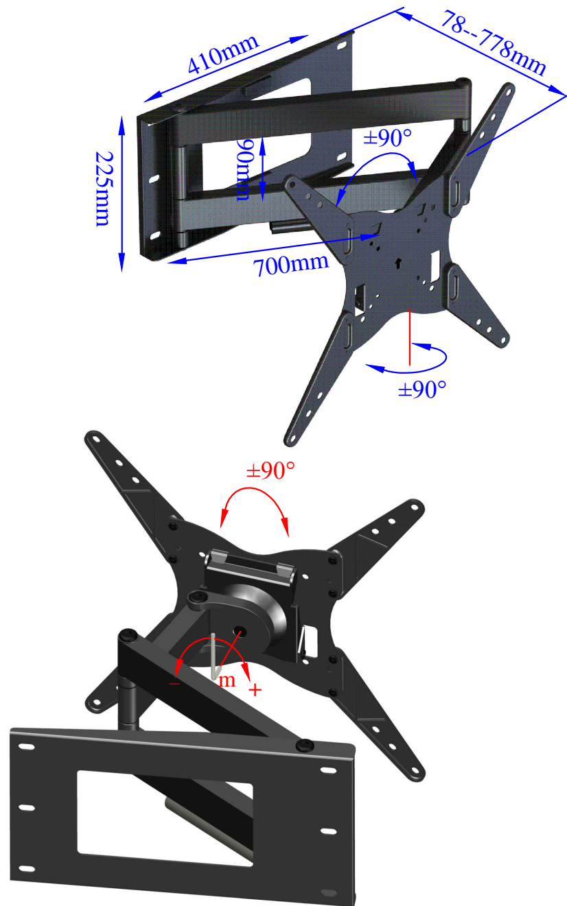
③ (VESA:300x300/400x400)
